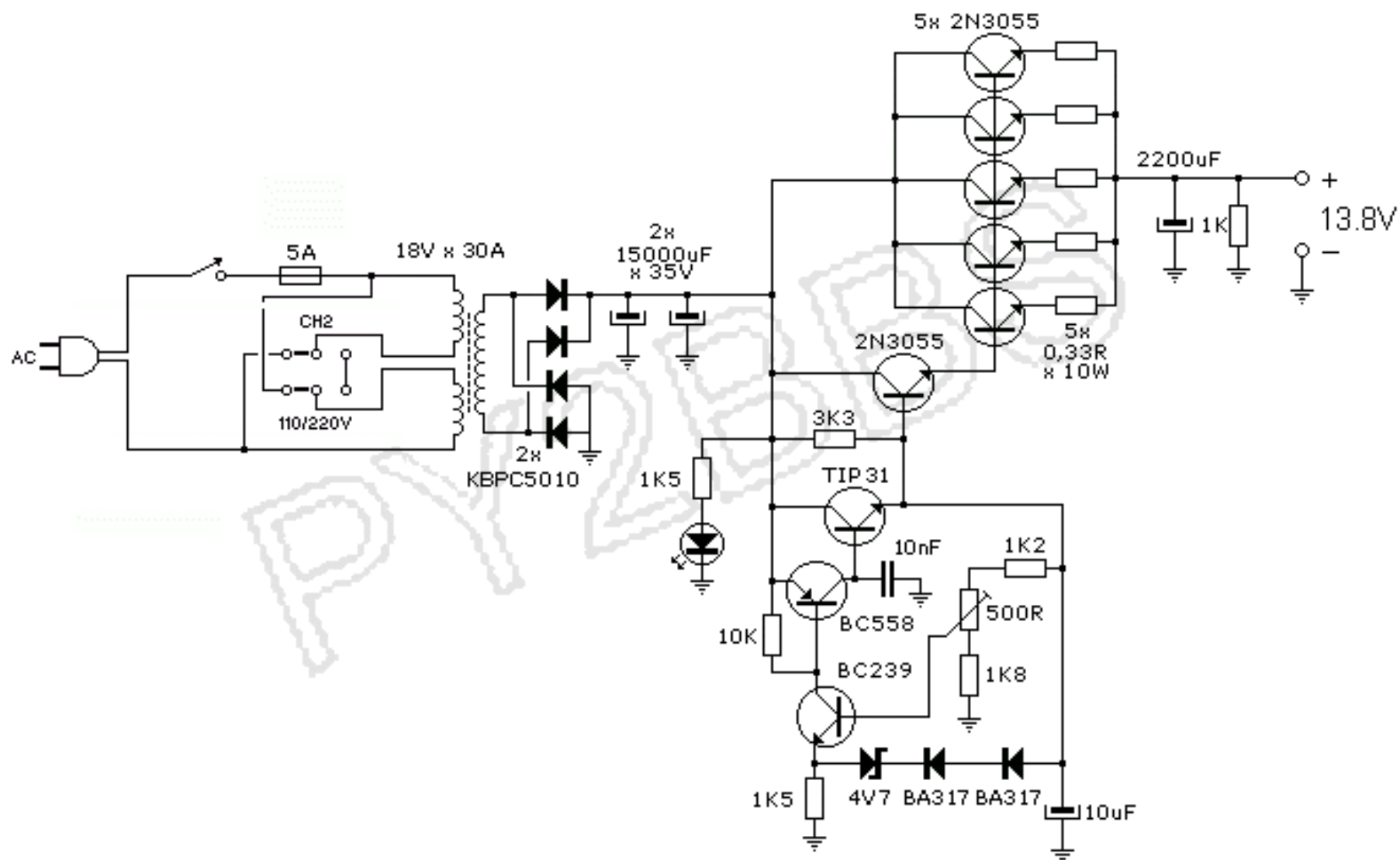
Fonte Soudy 30A modelo antigo
