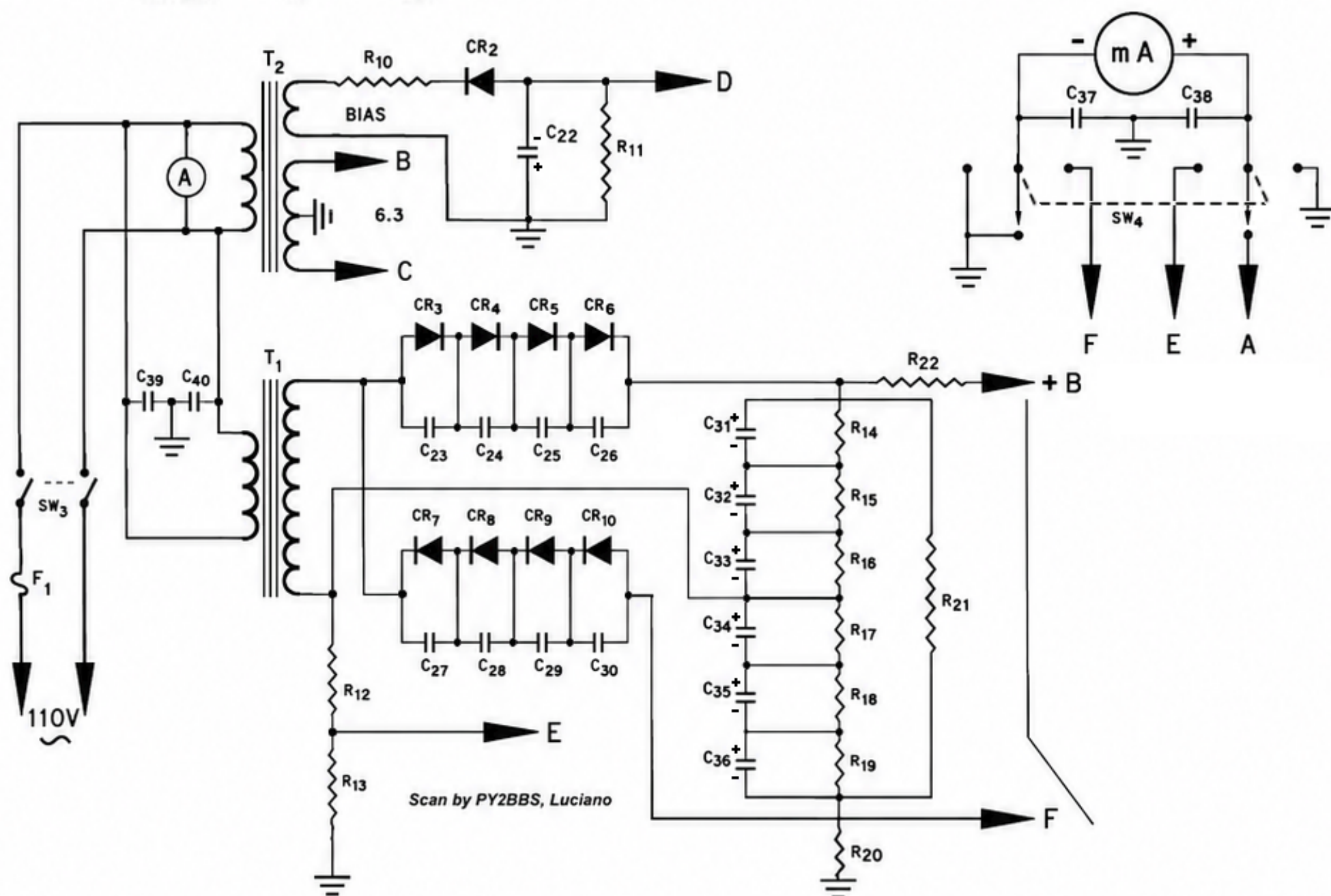
MARCOL Amplificador Linear - Mod. KW1
